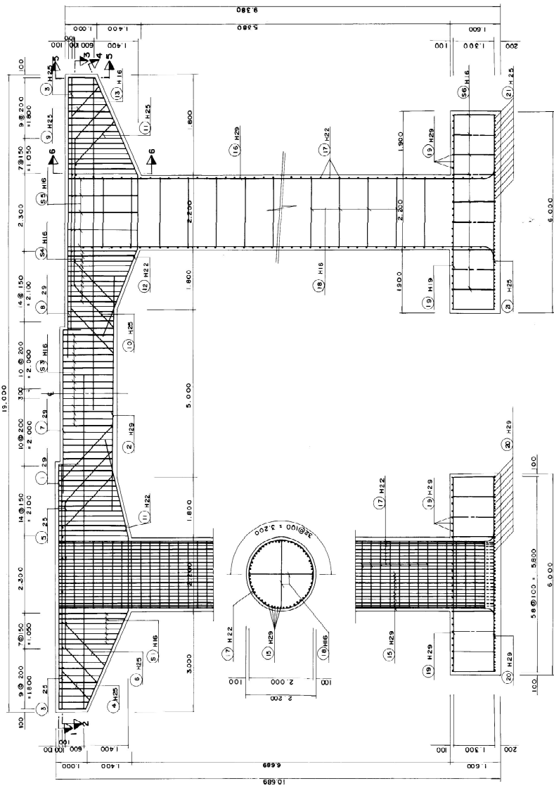
정면도 S=1:50
